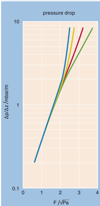
Mellapak 350.Y
