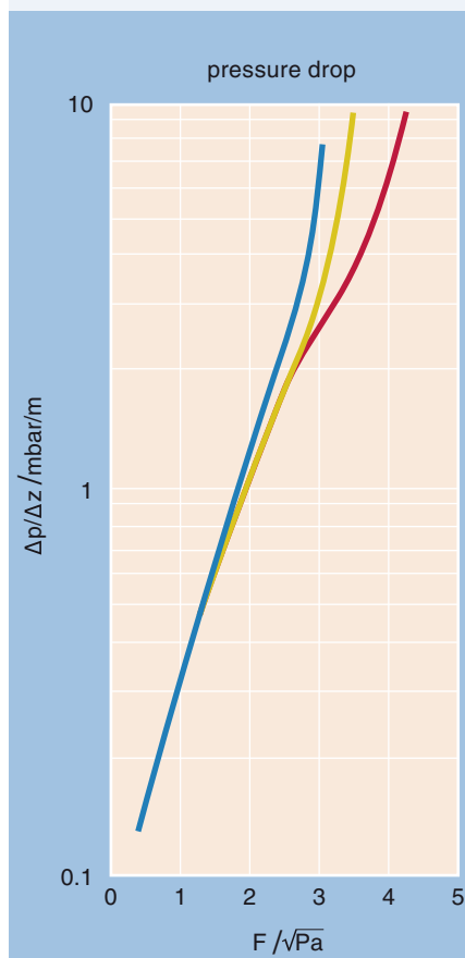
MellapakPlus 352.Y
