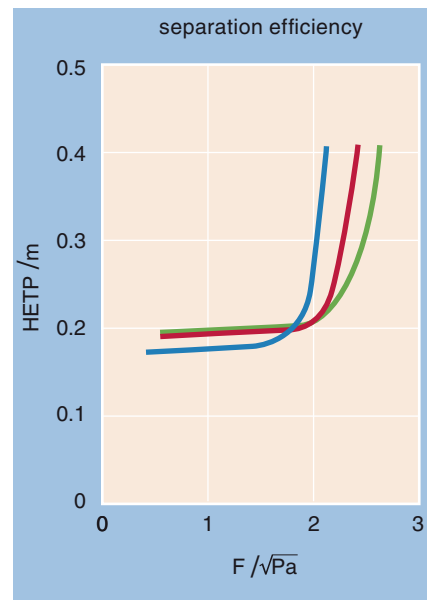
Mellapak 750.Y 960 ——— 100 ——— 50 ——— parameter = head pressure p /mbar
