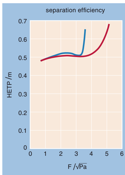
MellapakPlus 202.Y 960 ——— 100 ——— parameter = head pressure p /mbar
