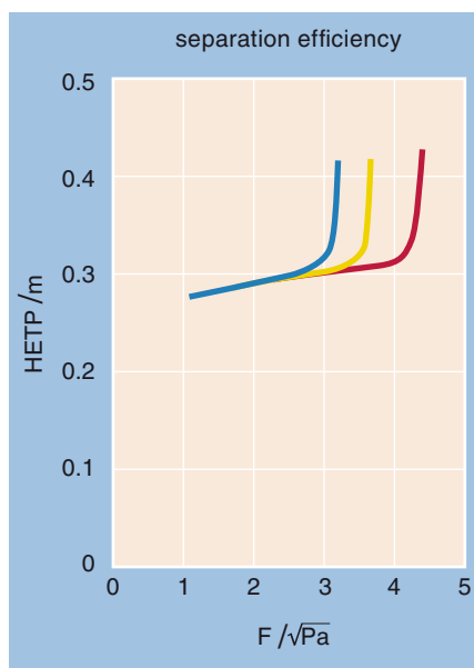
MellapakPlus 352.Y 960 ——— 400 ——— 100 ——— parameter = head pressure p /mbar
