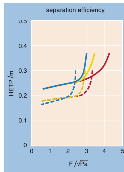
MellapakPlus 452.Y MellapakPlus 752.Y 960 ——— 960 - - - - 400 ——— 400 - - - - 100 ——— 100 - - - - parameter = head pressure p /mbar
