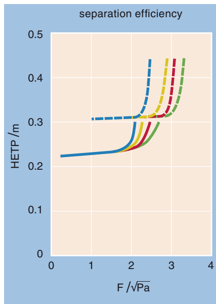
Mellapak 500.Y Mellapak 500.X 960 ——— 960 - - - 400 ——— 400 - - - 100 ——— 100 - - - 50 ——— 50 - - - parameter = head pressure p /mbar
