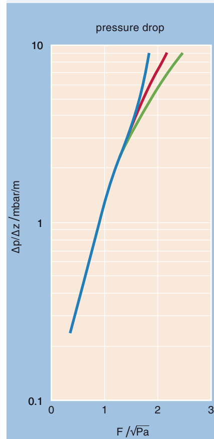
Mellapak 750.Y
