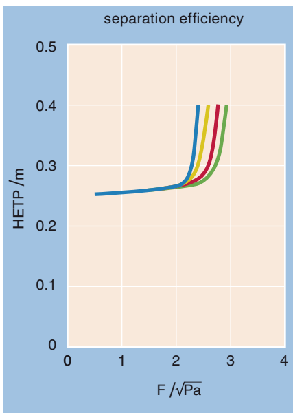
Mellapak 350.Y 960 ——— 400 ——— 100 ——— 50 ——— parameter = head pressure p /mbar
