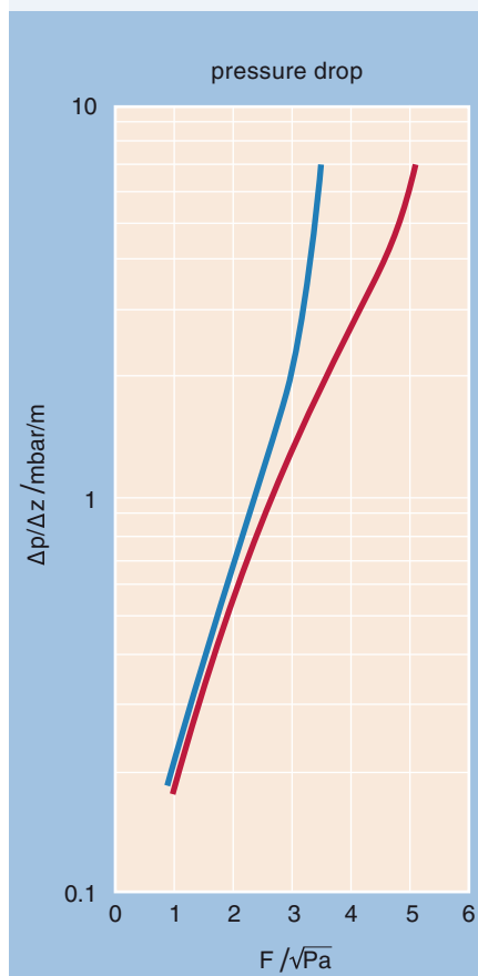
MellapakPlus 202.Y
